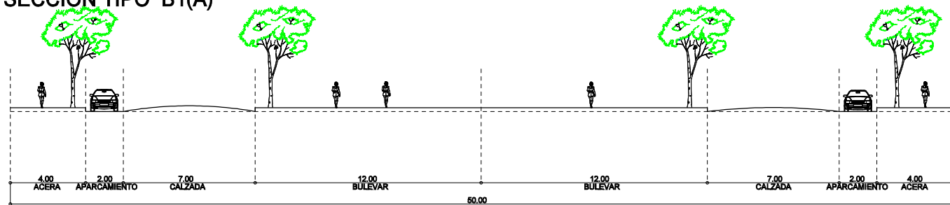
SECCION TIPO B1(A)
