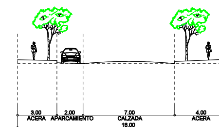
SECCION TIPO (F)
