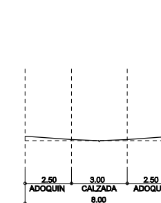
SECCION TIPO R3(K)
