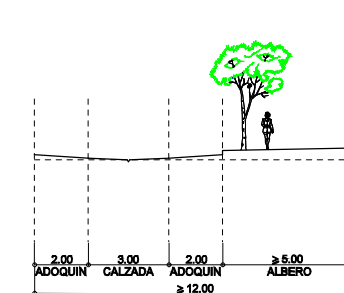
SECCION TIPO R3(J)
