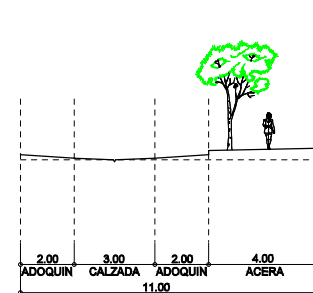
SECCION TIPO (I)
