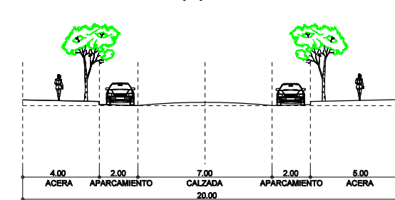
SECCION TIPO (E)
