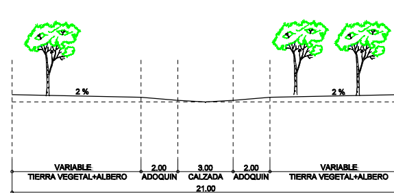
SECCION TIPO R1(C)
