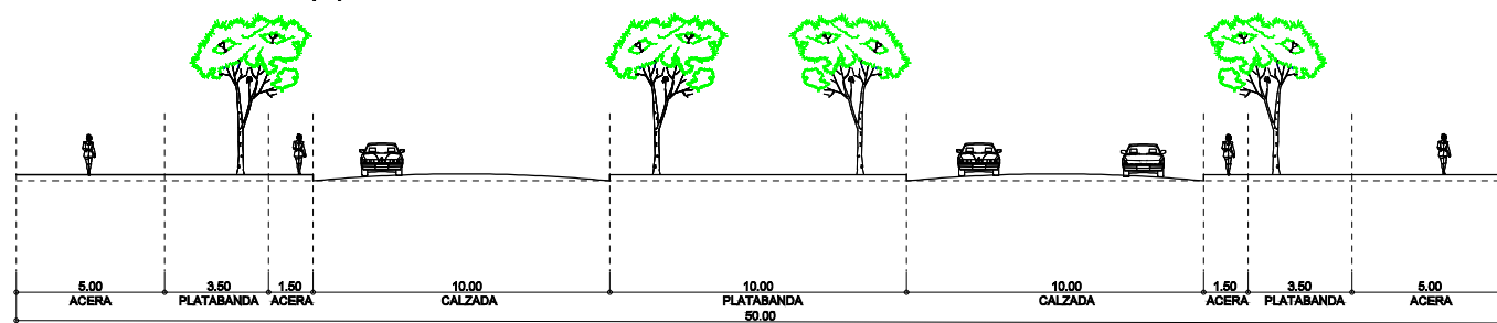
SECCION TIPO VP(B)
