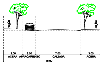
SECCION TIPO D2(H)
