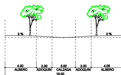
SECCION TIPO R2(G)
