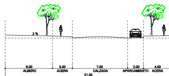
SECCION TIPO D1(D)
